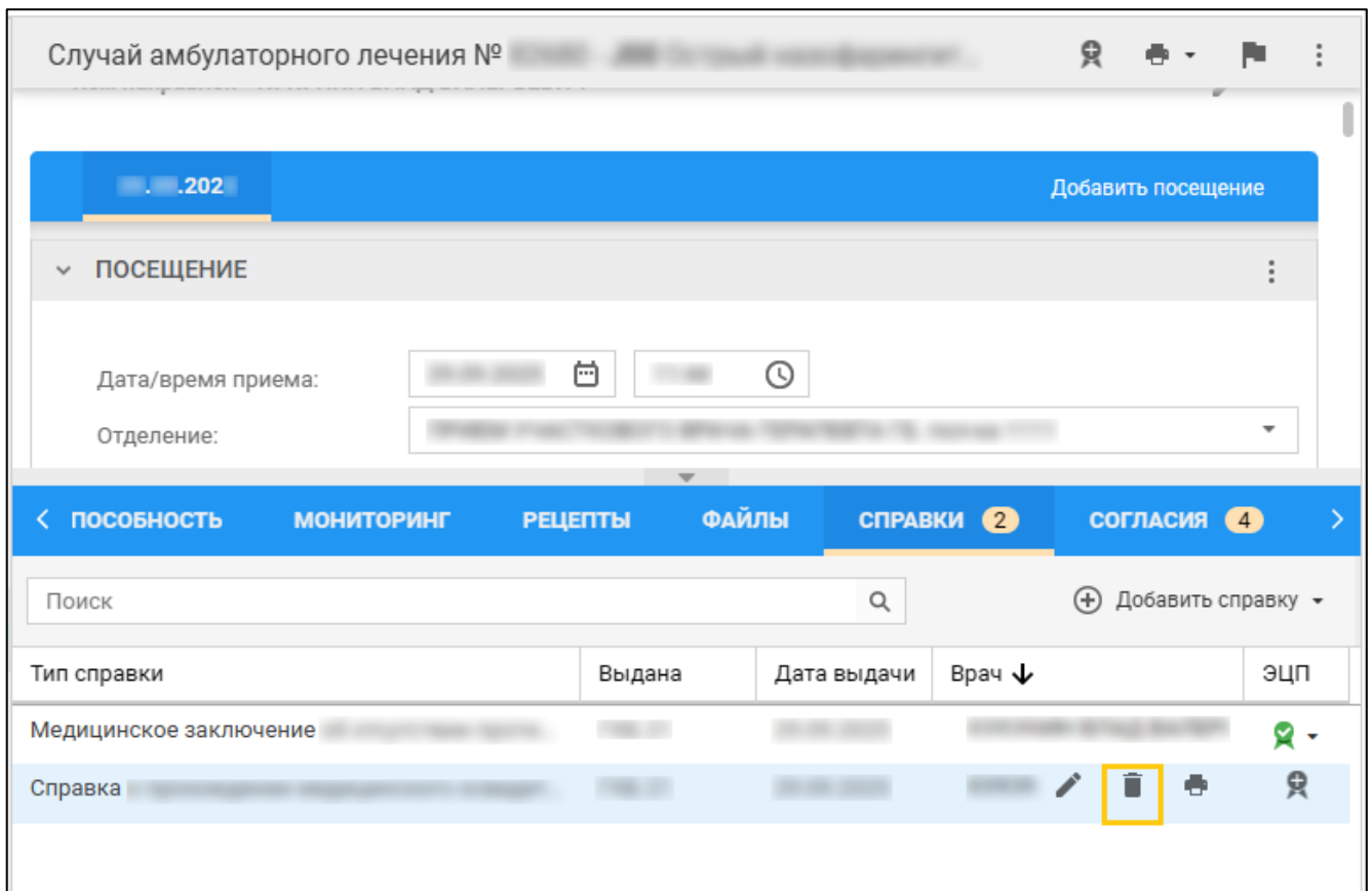
Рисунок 15 -- Удаление справки
